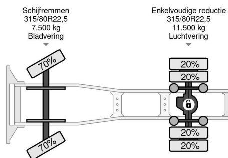
MAN 19.403 F2000 SLEEPERCAB (EURO 2 / ZF16 M... 4x2
